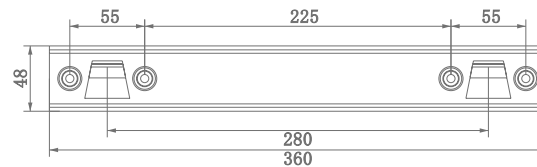
(挂板尺寸图，单位：mm)
