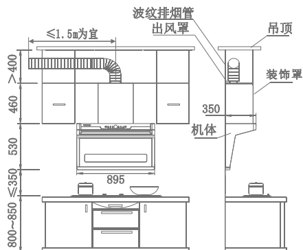
排烟管走橱柜安装示意图
