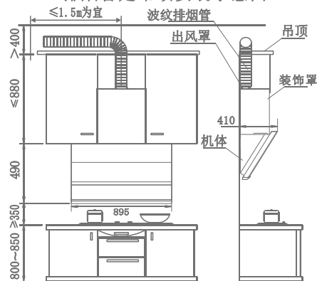
侧视图
