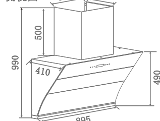
侧视图
