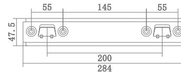
(挂板尺寸图，单位：mm)
