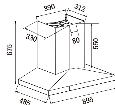
侧视图
