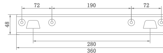
(挂板尺寸图，单位：mm)
