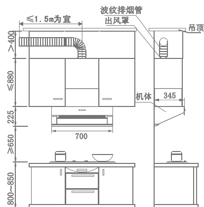
排烟管走橱柜安装示意图
