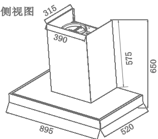
侧视图
