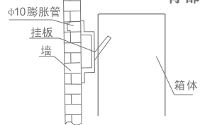
背部示意图
