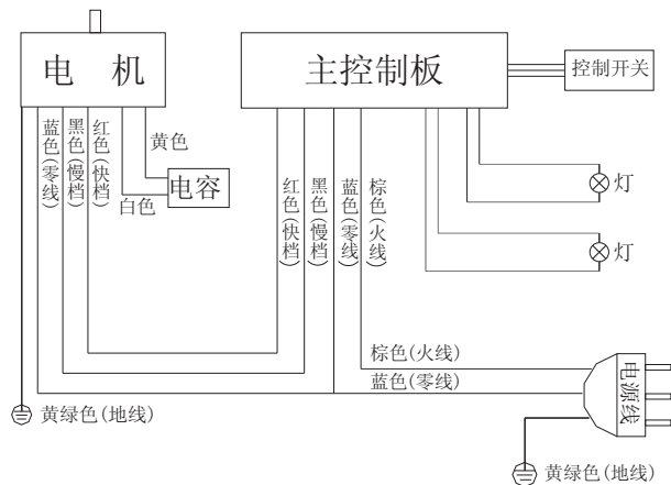
CXW-220-X7电器原理图
