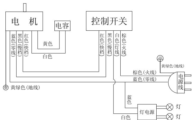
CXW-220-B39电路原理图
