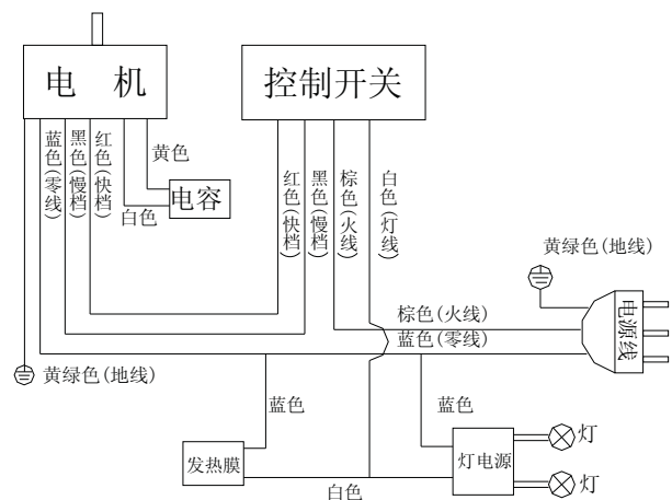
CXW-220-B36电路原理图
