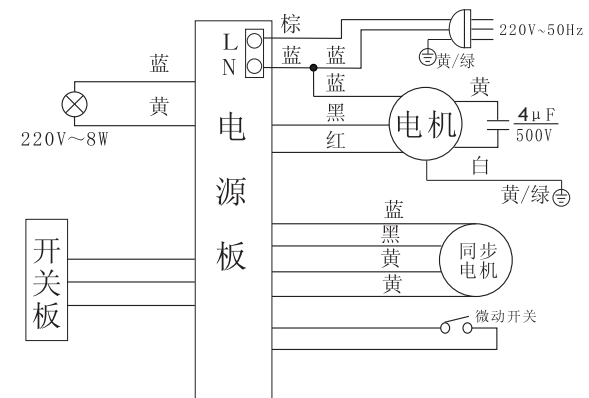
CXW-220-B28电路原理图
