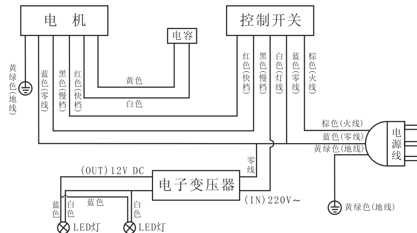
CXW-220-B3电路原理图
