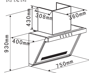
侧视图
