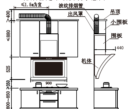
侧视图
