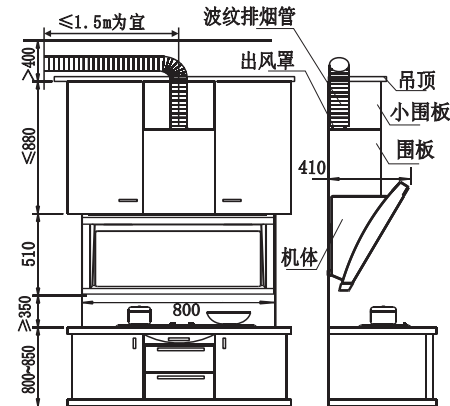
侧视图
