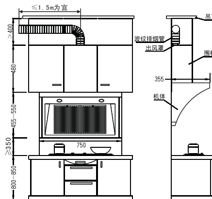
排烟管走橱柜安装示意图
