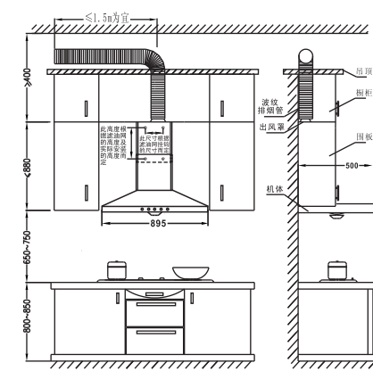
排烟管走吊顶安装示意图
