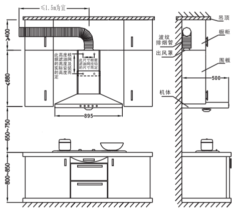
(图一)
