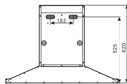
背面图
