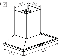
侧视图
