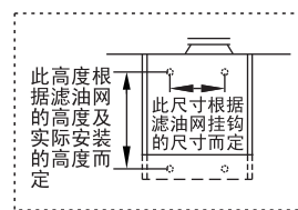
放大图
