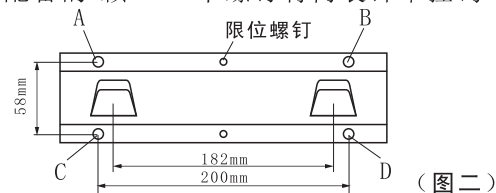
(图二)
