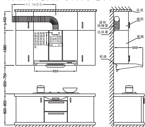
排烟管走橱柜安装示意图
