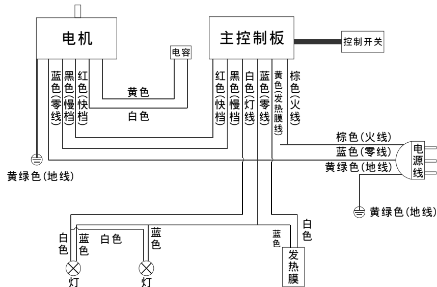
(CXW-220-A9电气原理图)
