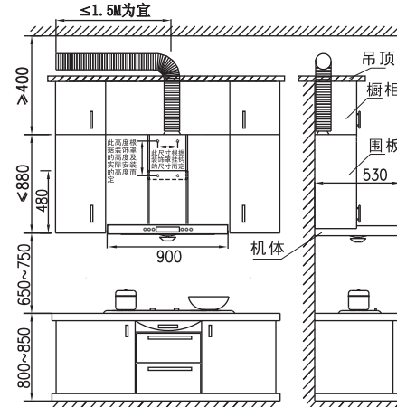
出风管走吊顶安装示意图
