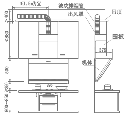
排烟管走吊顶安装示意图
