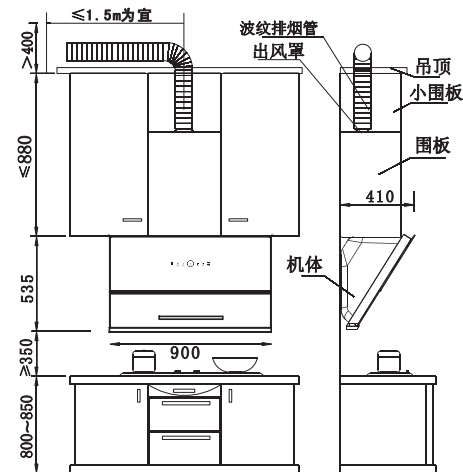
侧视图
