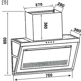
侧视图
