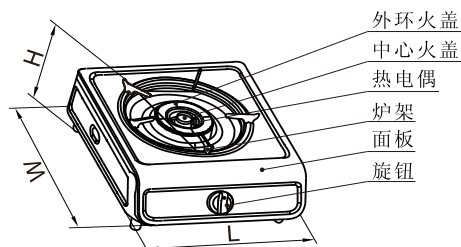
图1：台式单眼灶
