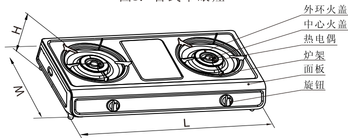
图2：台式双眼灶
