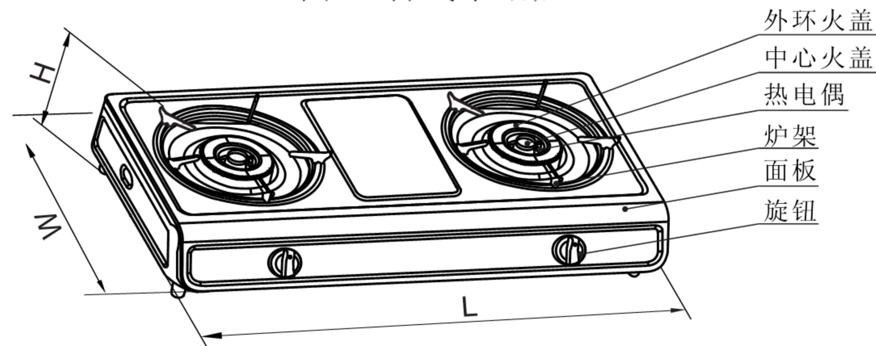
图2：台式双眼灶
