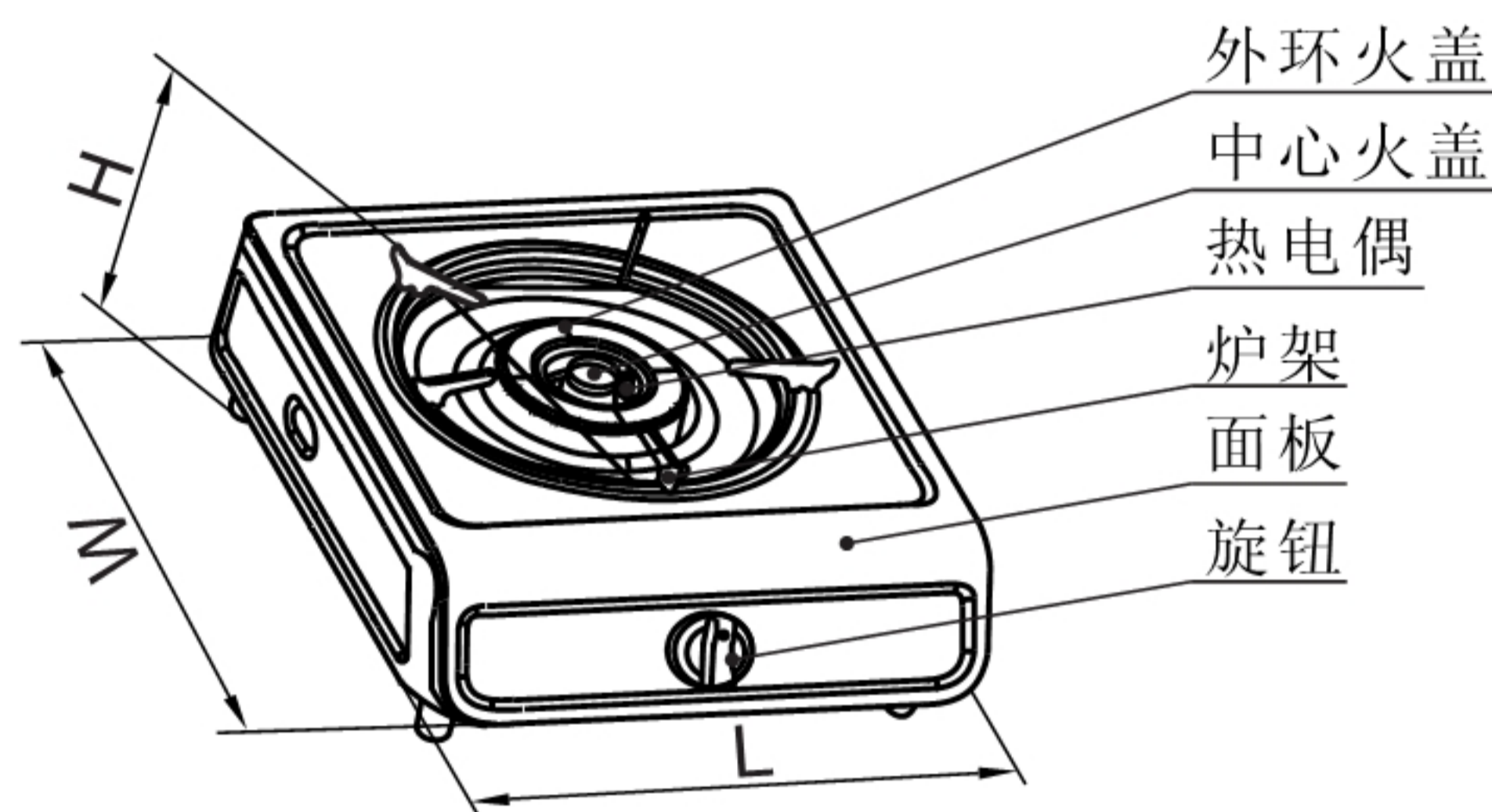
图1：台式单眼灶
