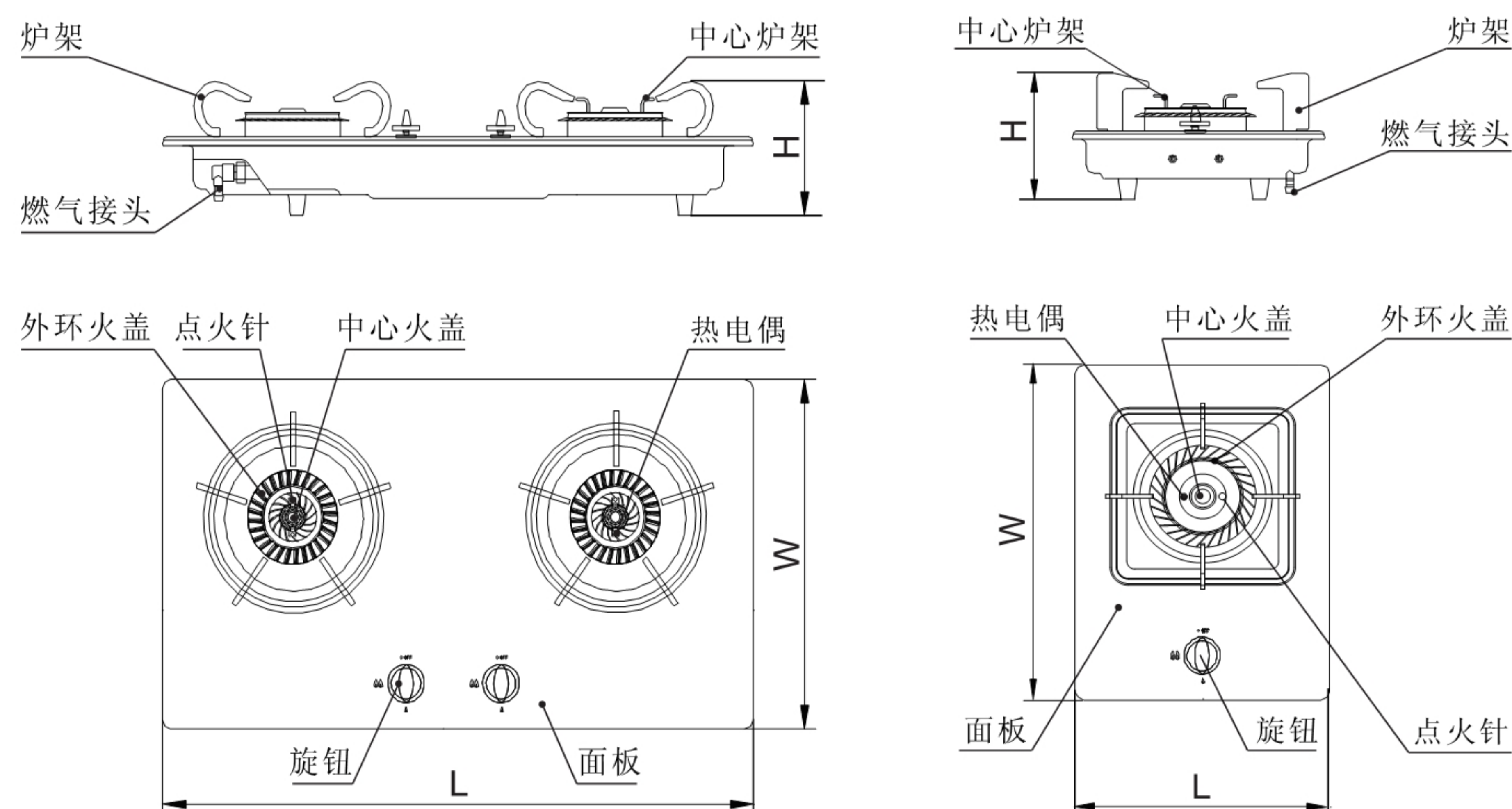
图1：嵌入式双灶
